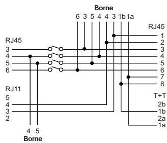
Schéma i (cavalier OFF)
